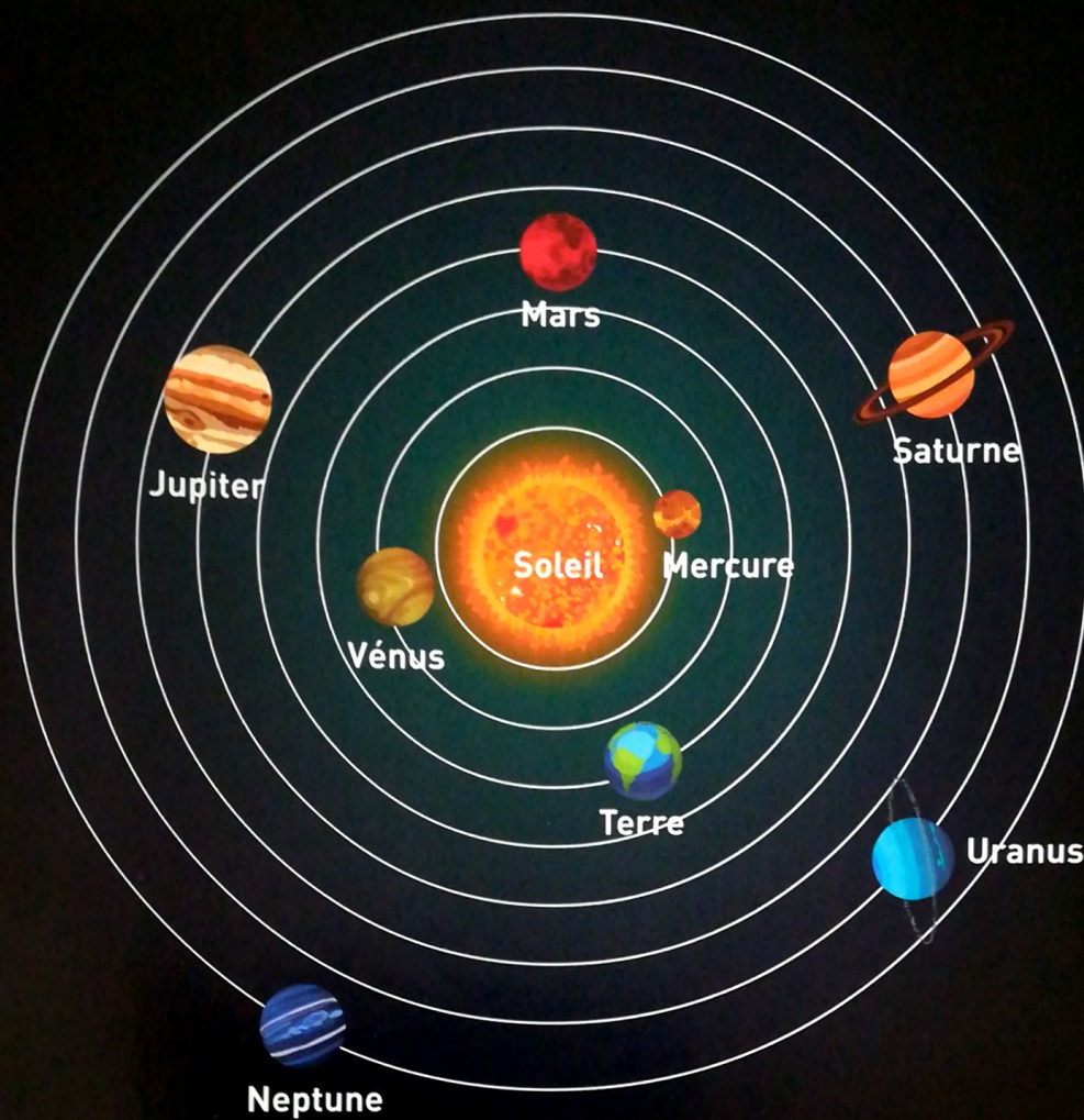
Le schéma du système solaire
